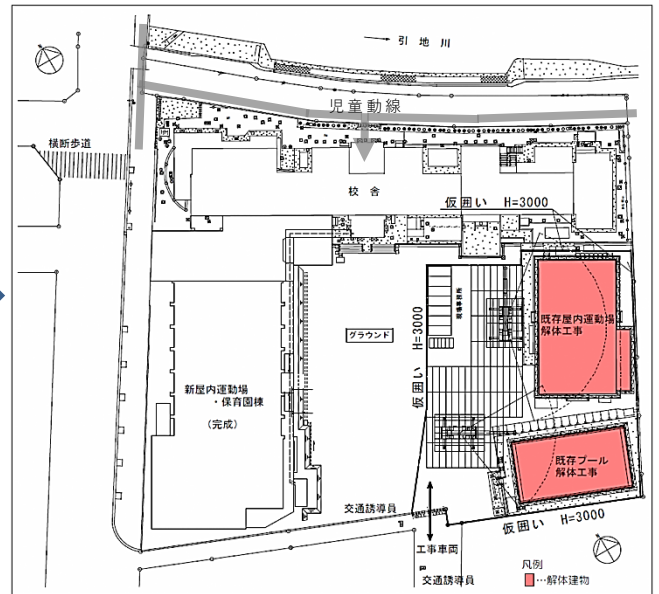
既存屋内運動場・プール等解体工事
