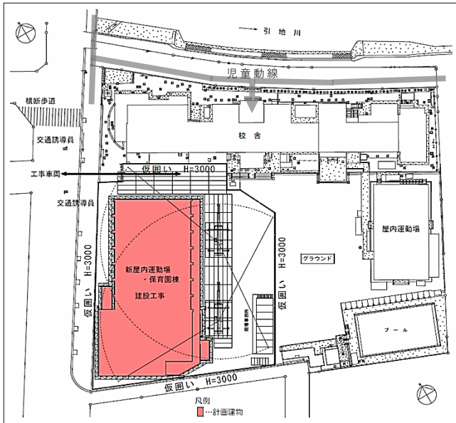
新屋内運動場・保育園建設工事
