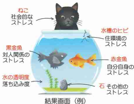
結果画面 (例)
