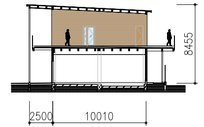
C棟断面图
