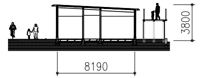
B棟断面图
