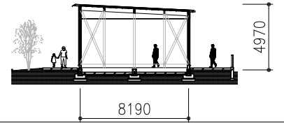
B棟断面图
