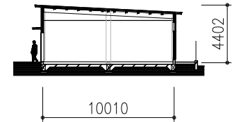
D棟断面图
