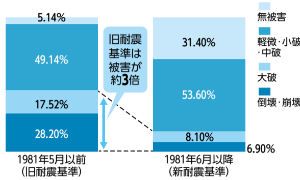
〔建築時期による木造住宅の被害状況 熊本地震の震源に近い益城町〕 日本建築学会
