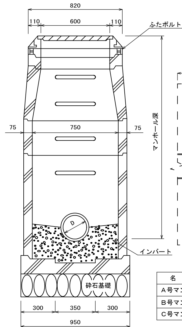
横断面図
