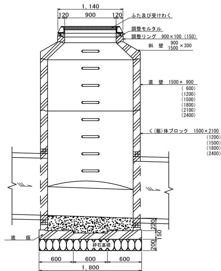
縦断面図
