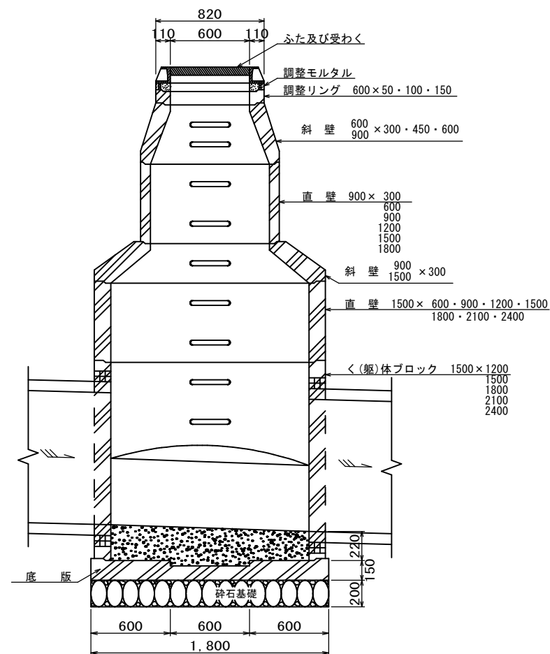
縦断面図
