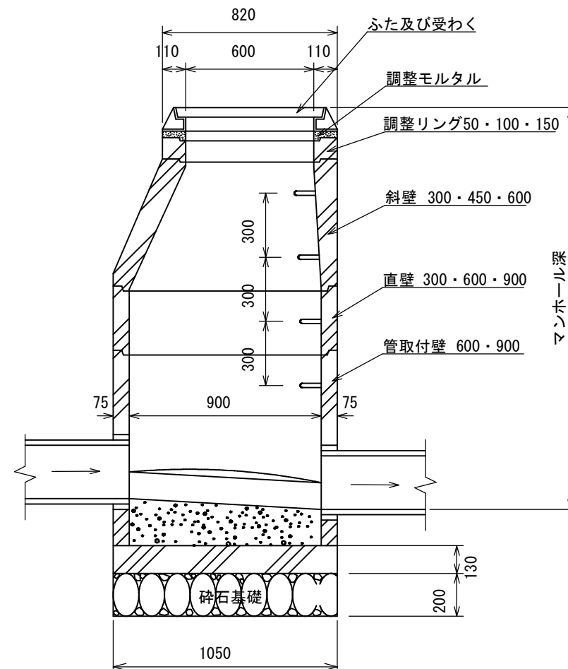
縦断面図
