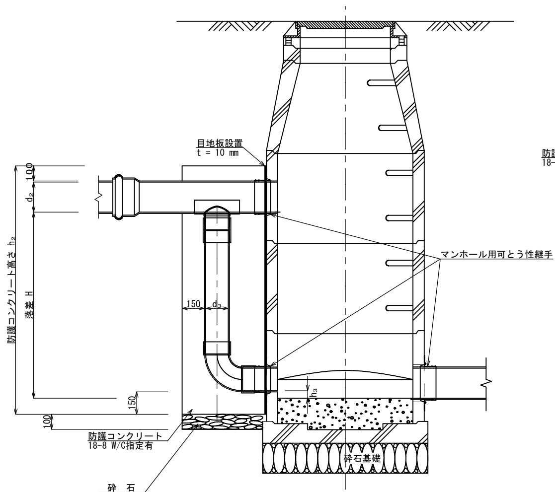
断面図
