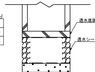
雨水ます（藤沢市B型）数量表（粘性土） 1基当たり
