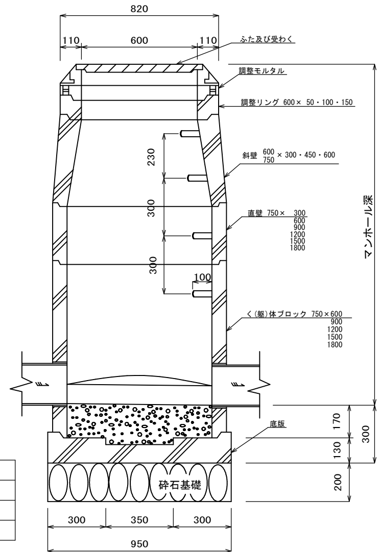
縦断面図
