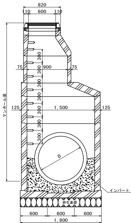
横断面図
