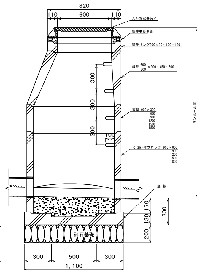
縦断面図
