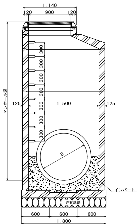
横断面図
