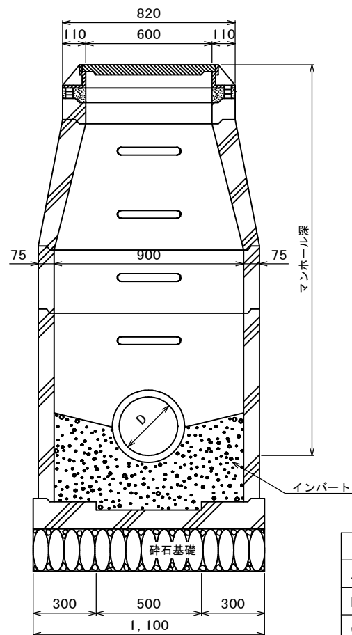
横断面図
