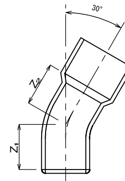
30° 曲管寸法
