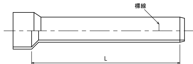
接着受口片受け直管寸法
