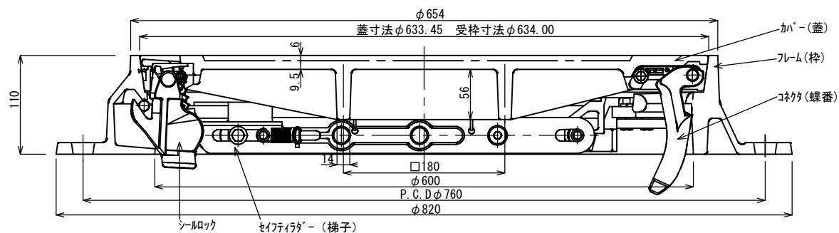
カバ-、フレーム断面図
