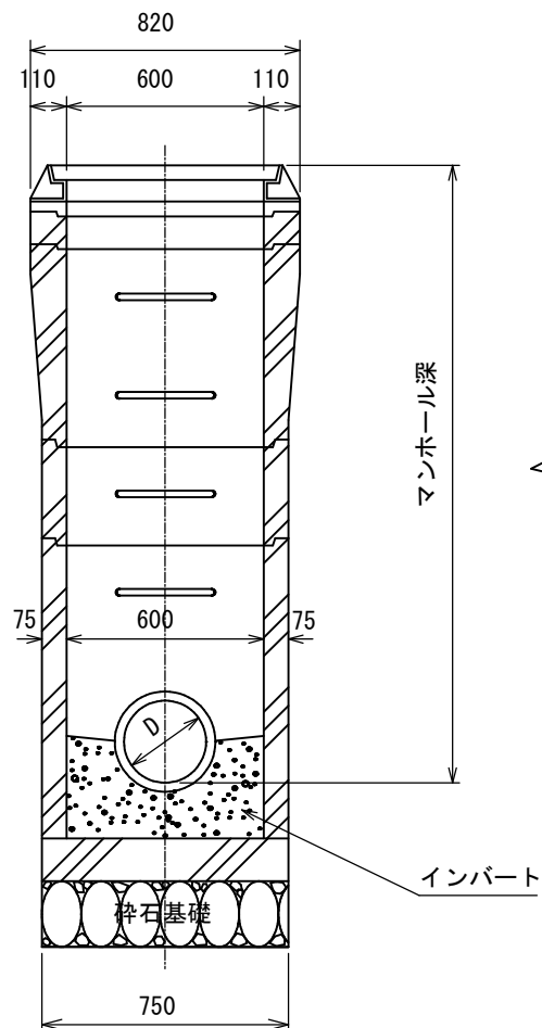
横断面図
