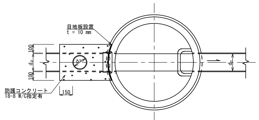
平面図
