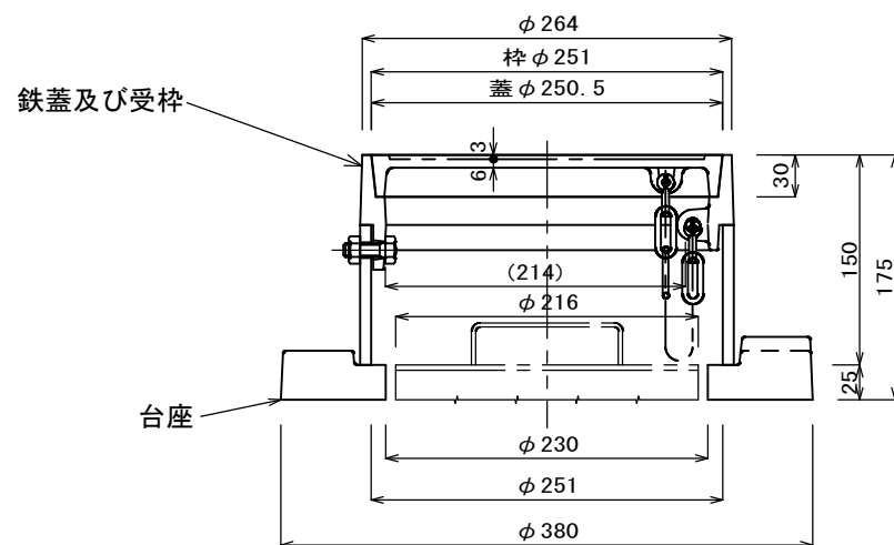
汚 水
