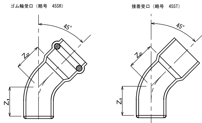
45° 曲管寸法
