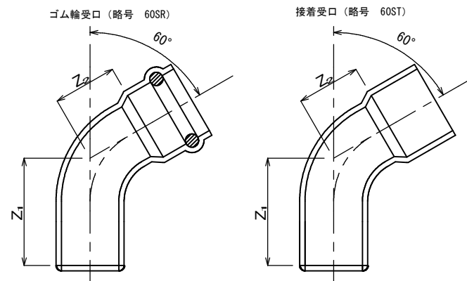
60° 曲管寸法
