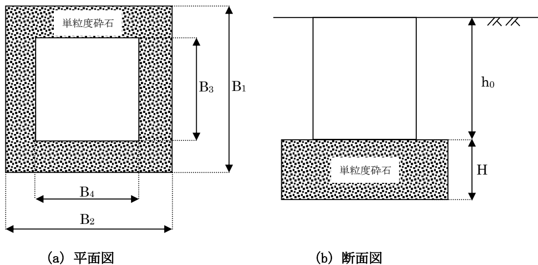
図 4-2-2 浸透枿 (底面浸透タイプ (置換材角型・角型枿))
