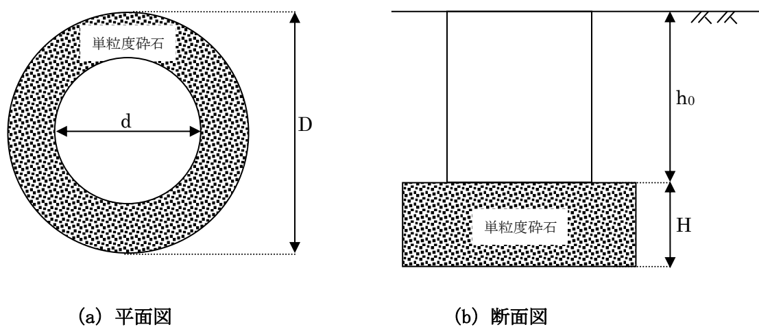
図 4-2-5 浸透樹（底面浸透タイプ（置換材円型・円型樹））
