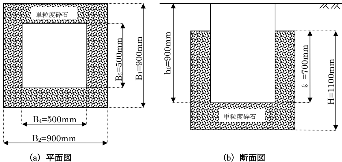
図 4-3-2 設置浸透枳断面図
