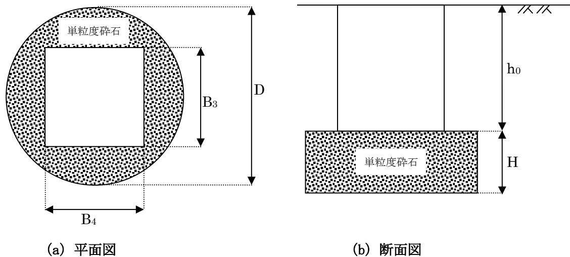
図 4-2-4 浸透樹（底面浸透タイプ（置換材円型・円型樹））
