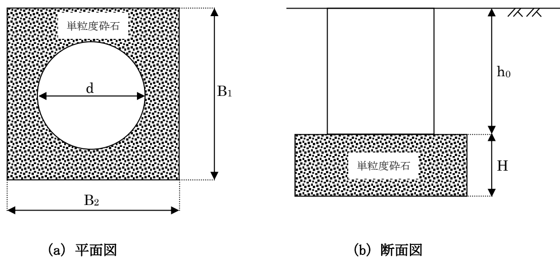
図 4-2-3 浸透枿 (底面浸透タイプ (置換材角型・円型枿))
