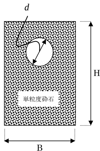
図 4-2-1 浸透管断面図
