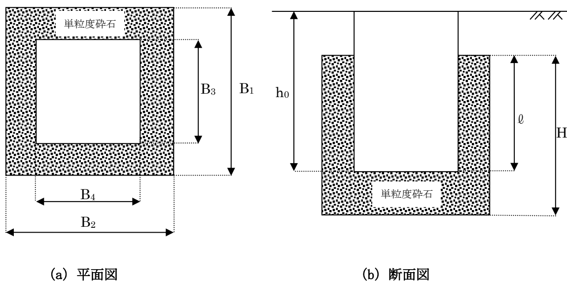
図 4-2-6 浸透櫛 (置換材角型・角型櫛)
