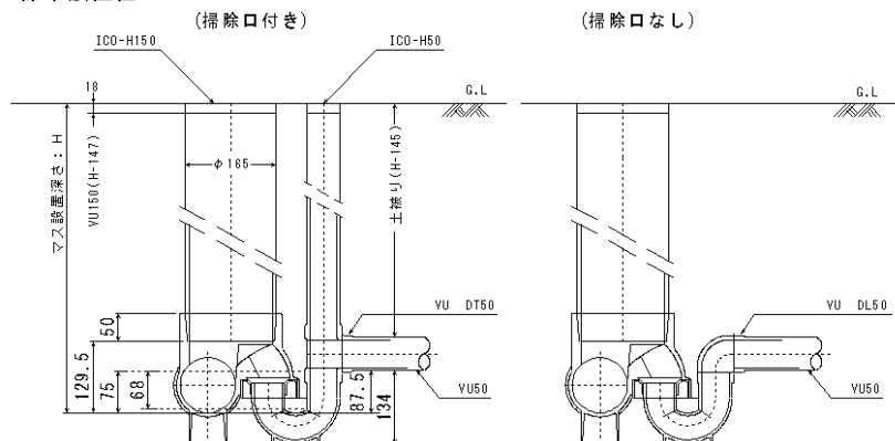
標準設置図
