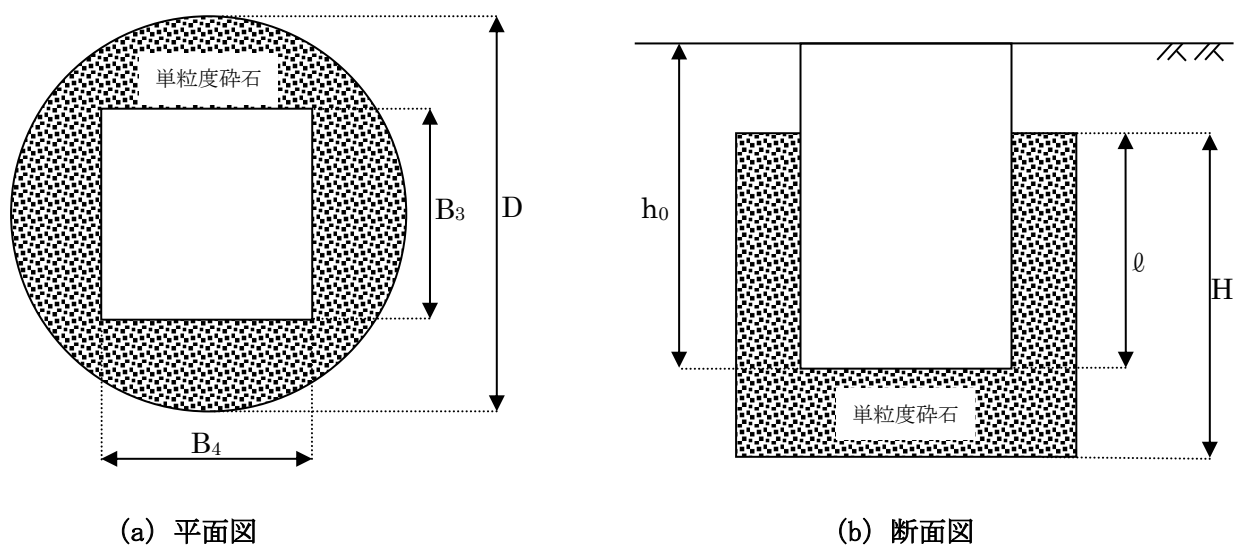
图 4-2-8 浸透柵（置換材円型・角型柵）
