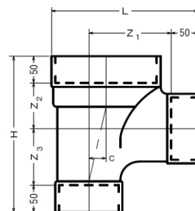
コウバイ 2/100
