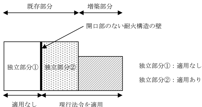
図 87-1 政令第 117 条第 2 項に該当する独立部分の例
