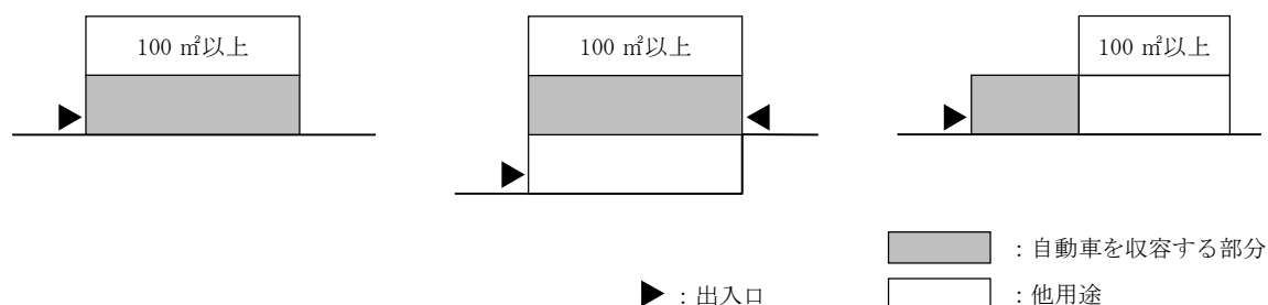
図 52-3 自動車を收容する部分のある階の直上階の床面積が100平方メートル以上のもの（第3号）
