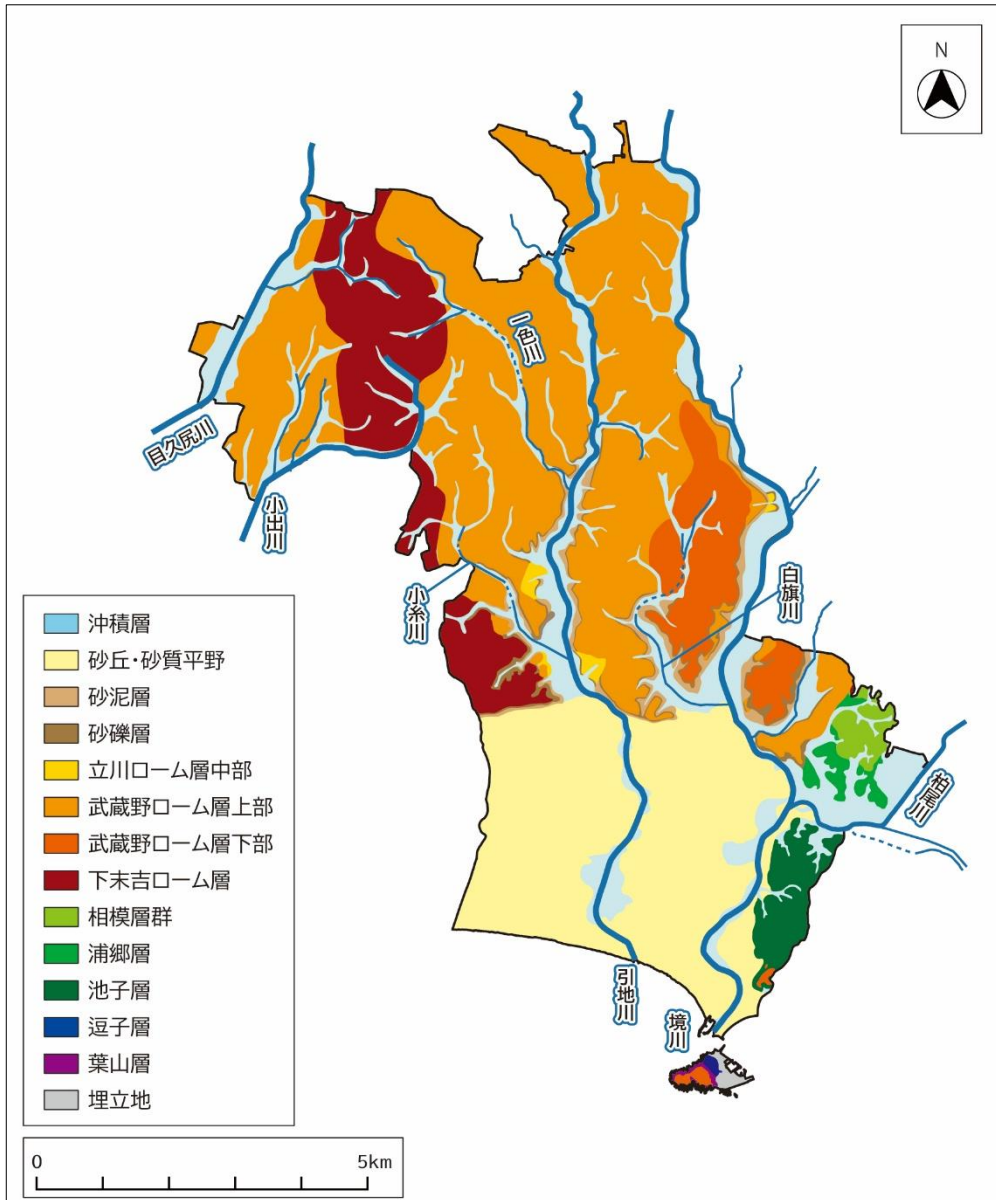
図5 地質図 (国土数値情報〔行政区画、河川〕を加工して作成)
