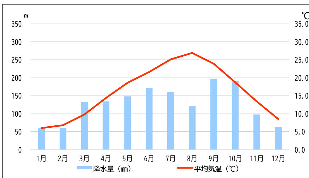
図7 雨温図（気象庁HP：1992～2020年の平年値より作成）
