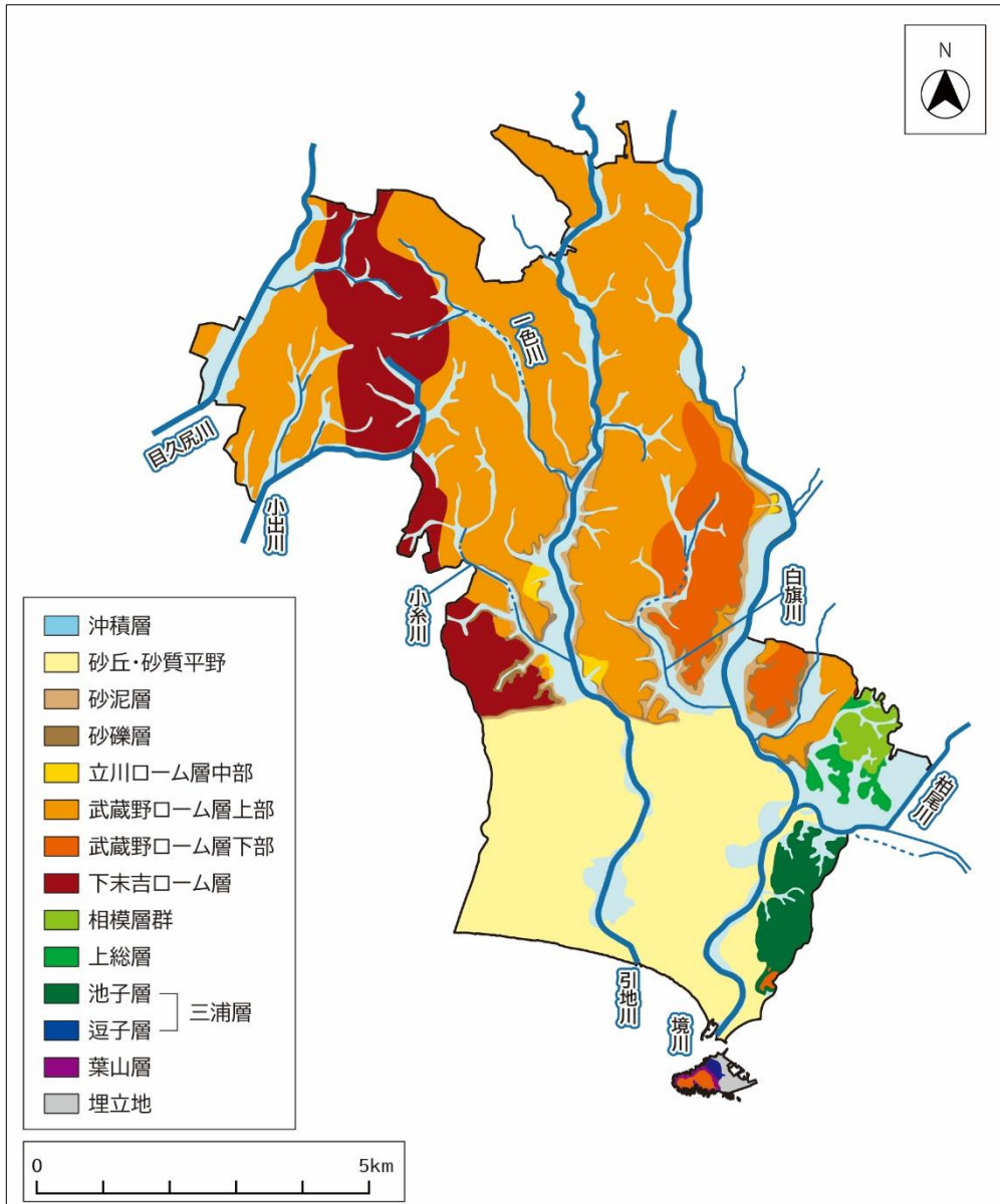
図5 地質図
