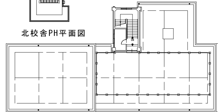
北校舎屋上平面図
