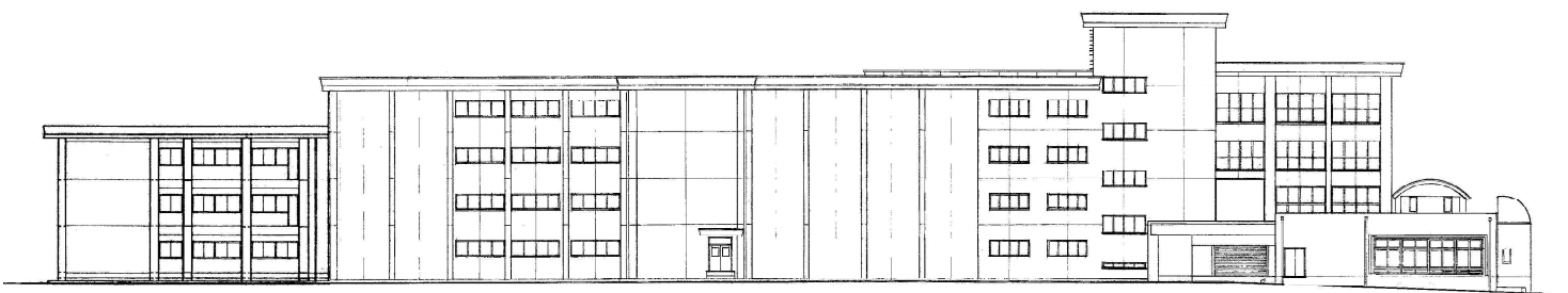
北立面图
