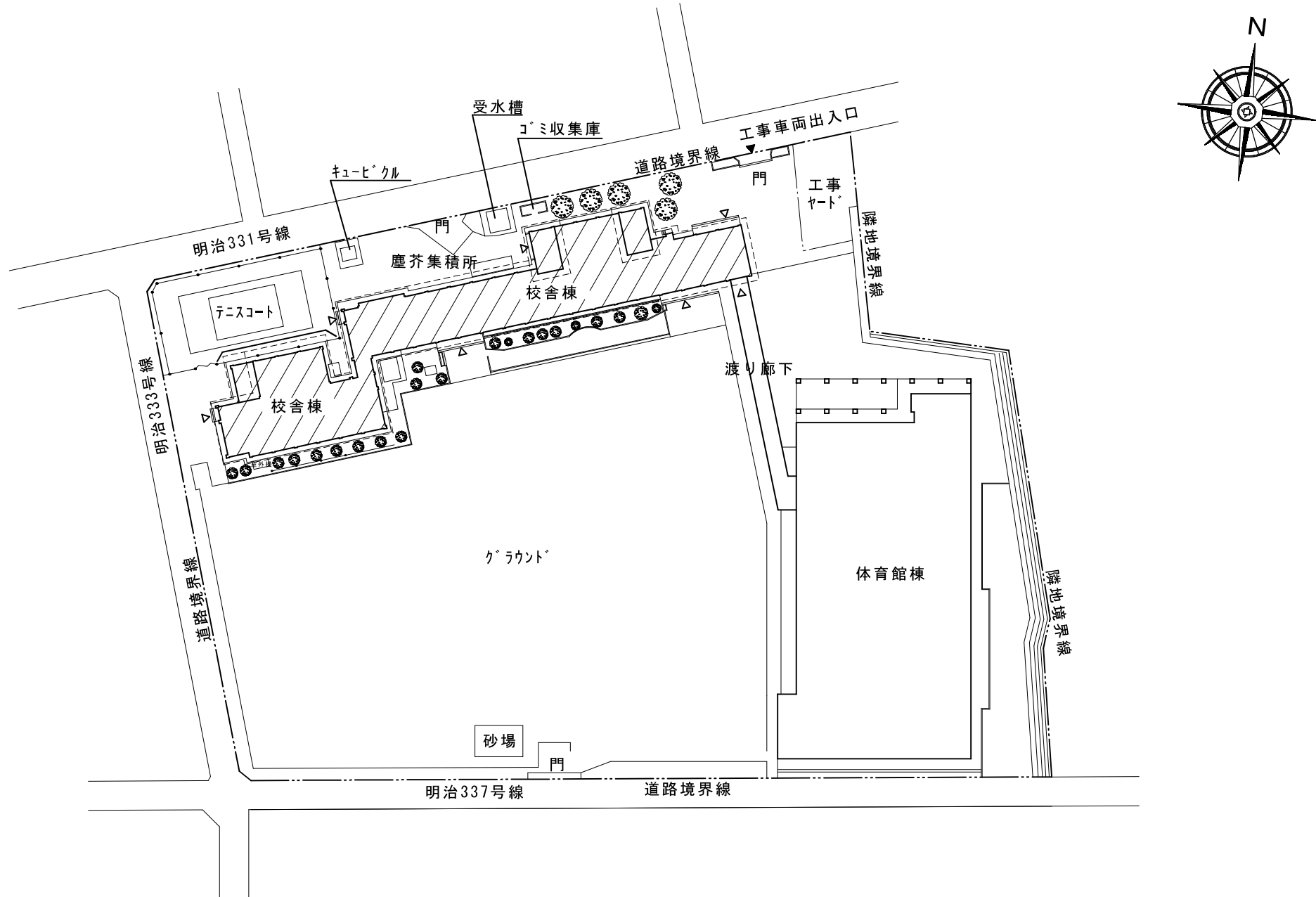
配置図 1/1000
