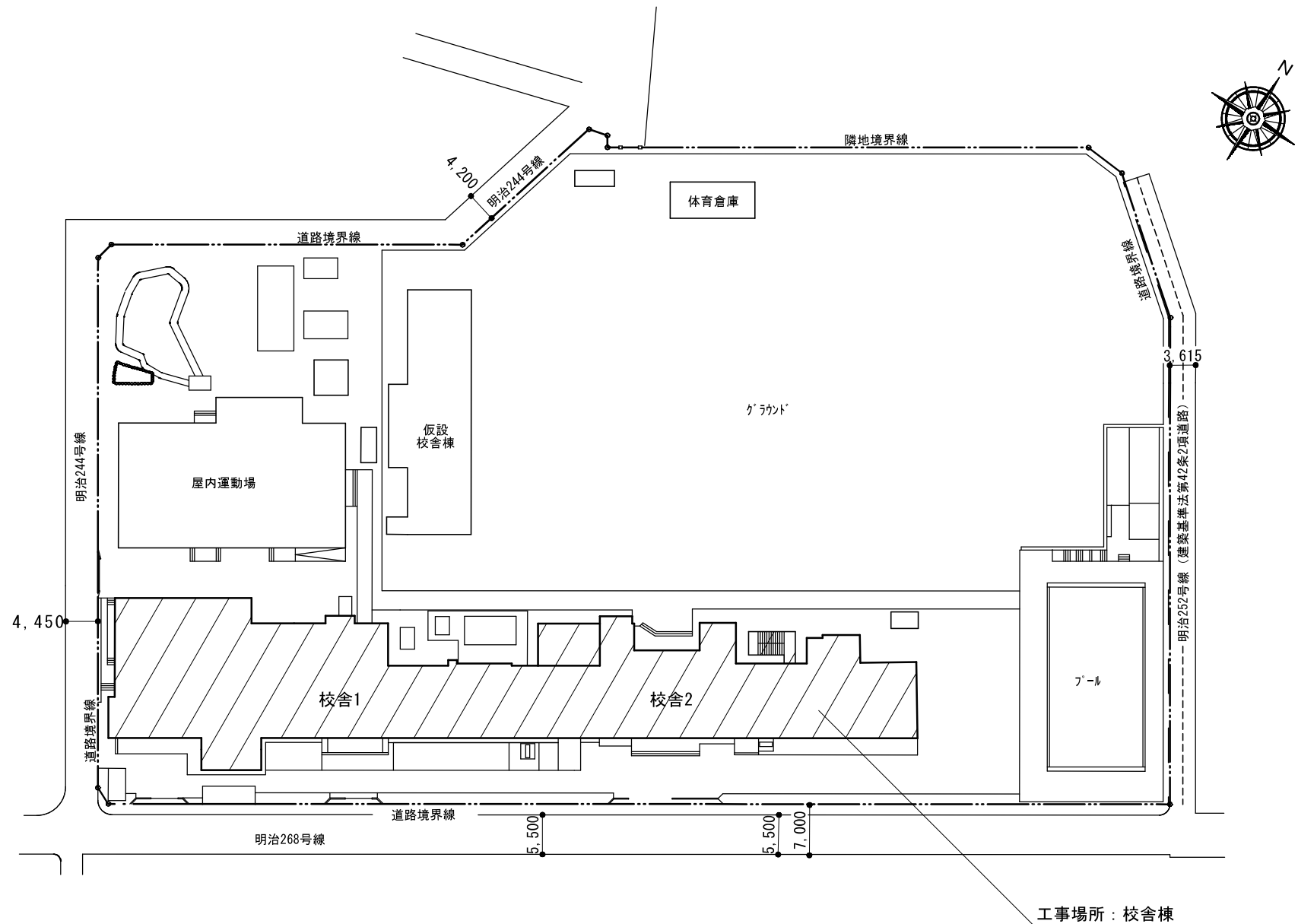
配置図 1/800
