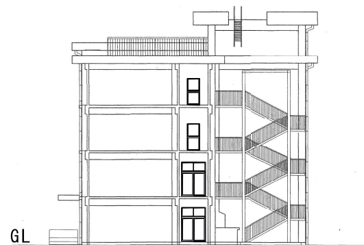
東立面图
