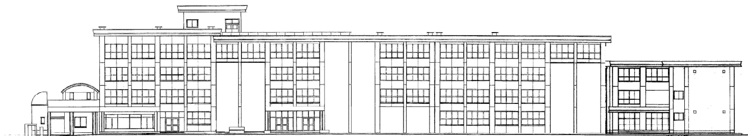
南立面图
