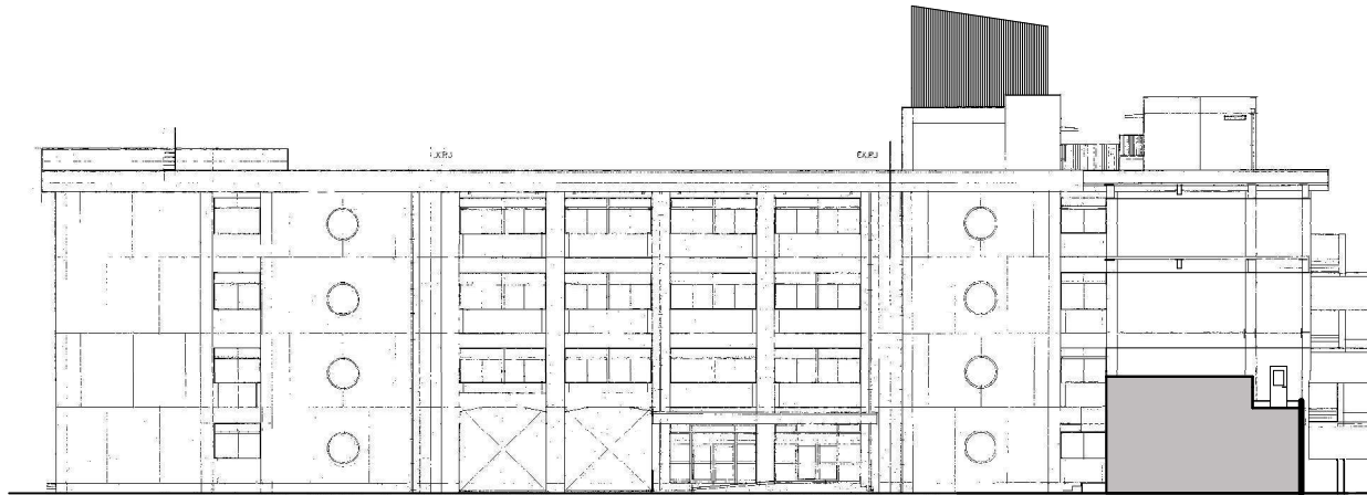
東立面図（校舎棟）
