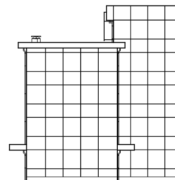
東側立面図③ 1/400
