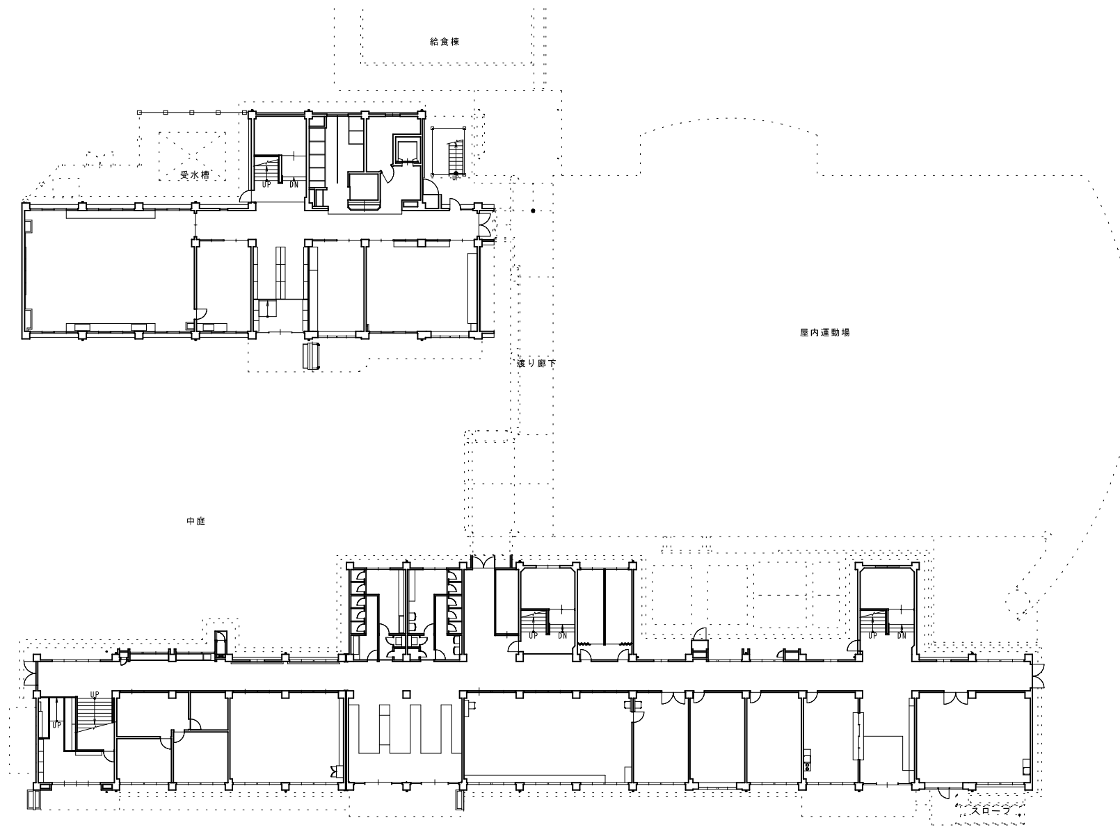
1階平面図 1/400
