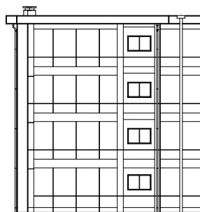
東側立面図② 1/400
