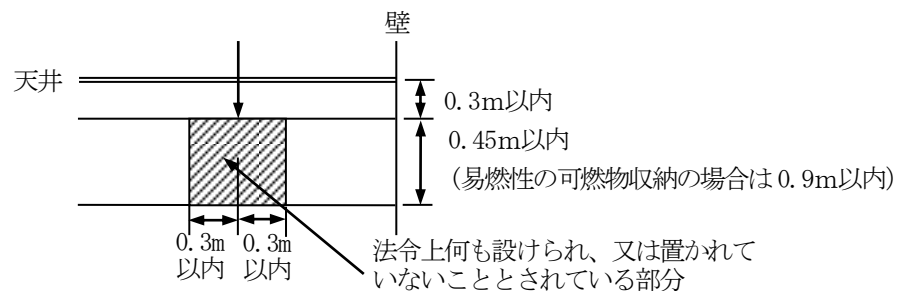
〔標準型ヘッド(小区画ヘッドを除く。): 断面〕
