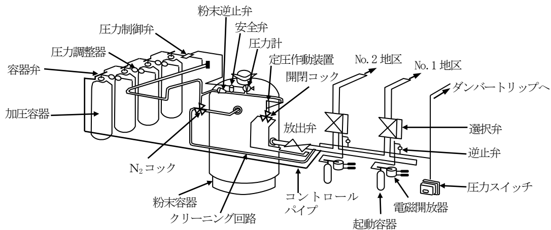
資料 粉末消火設備粉末容器附属機器図
