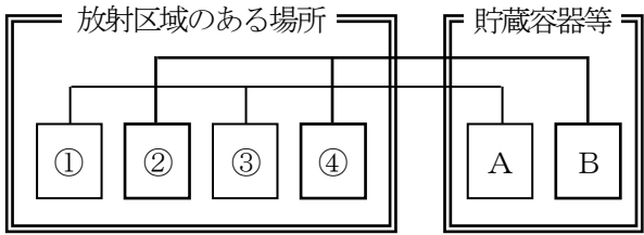
第 7－1 図 直列の放射区域ごとの貯蔵容器等の組み合わせ例
