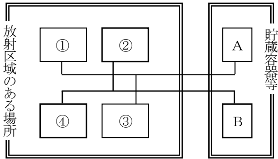
第 7－2 図 並列の放射区域ごとの貯蔵容器等の組み合わせ例
