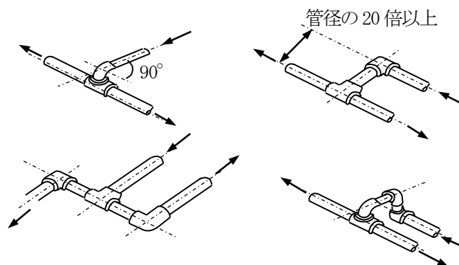
別図第 7-2 粉末消火設備における T 型継手の良い配管方法
