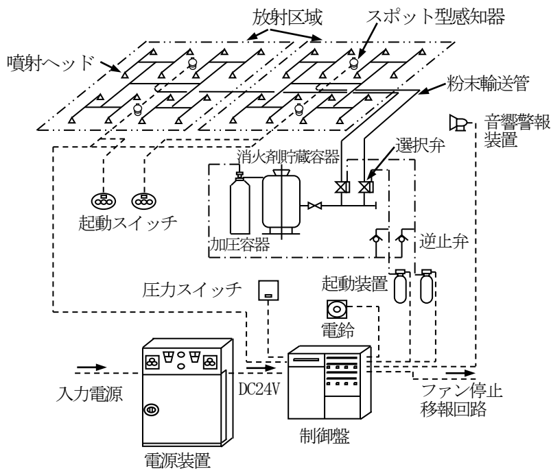
別図第 7-1 粉末消火設備系統図
