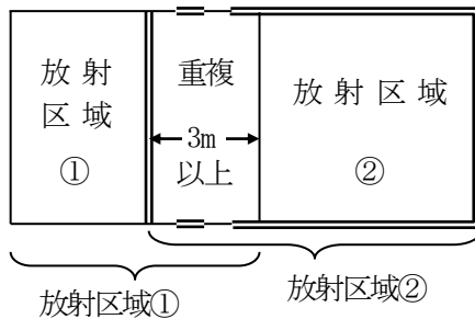
第7－4図 2放射区域のみで3m以上の重複がある場合の消火剤の貯蔵量の例
