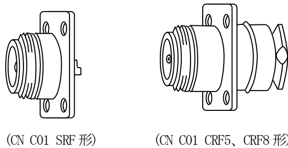
第22-1図 JIS C5411 C01形コネクタ外観図
