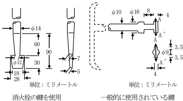
第22-2図 鍵の形状
