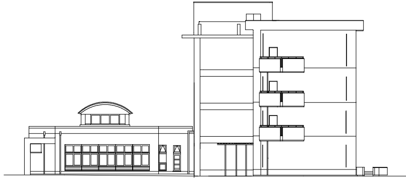
西立面図
