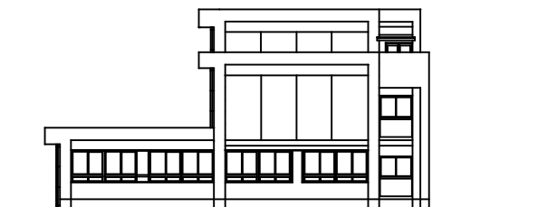
西立面図
