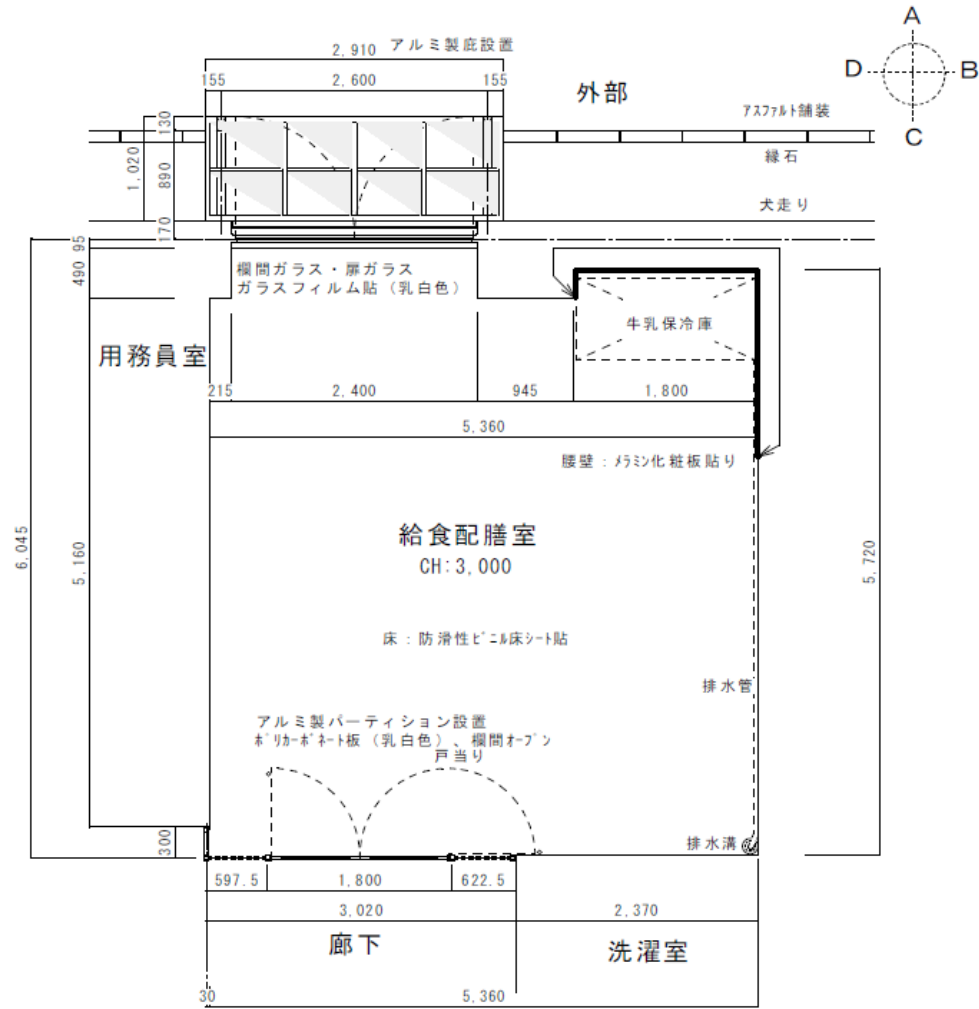
給食配膳室 平面図
