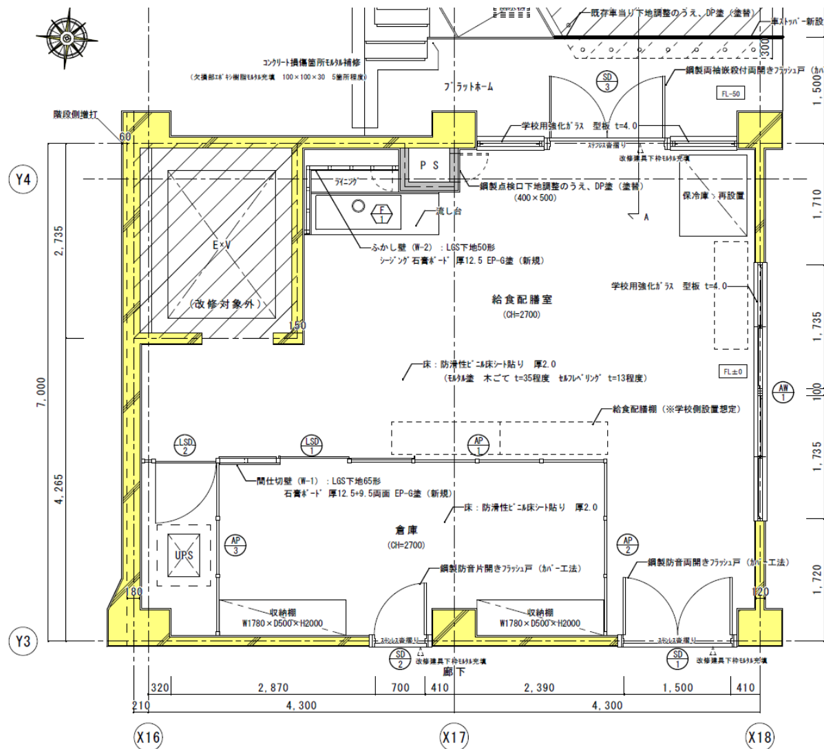
配膳室改修後詳細平面図 1/50
