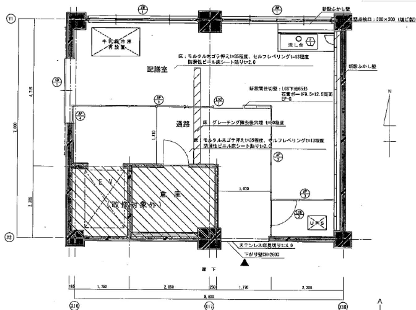
配膳室改修後平面図 1/50
