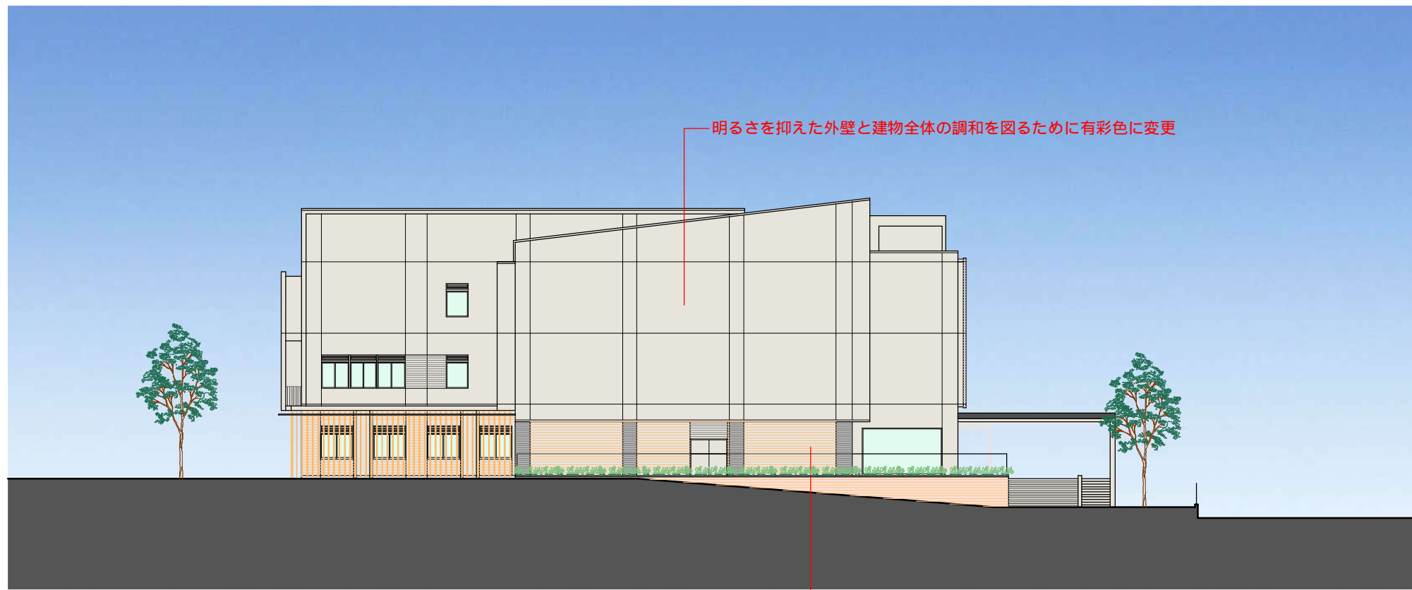
西立面図 1:300
